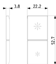
Vista ingombri
