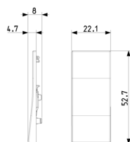
Vista ingombri
