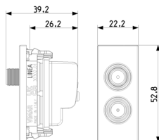
Vista ingombri
