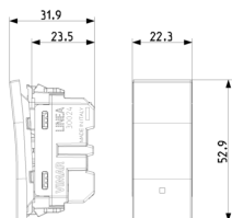
Vista ingombri
