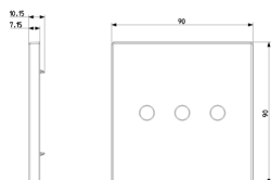
Vista ingombri
