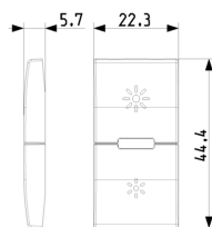
Vista ingombri
