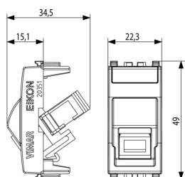
Vista ingombri
