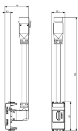
Vista ingombri
