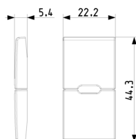
Vista ingombri
