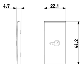
Vista ingombri
