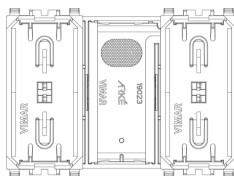
Vista posteriore
