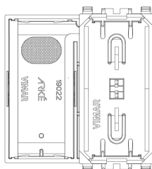
Vista posteriore
