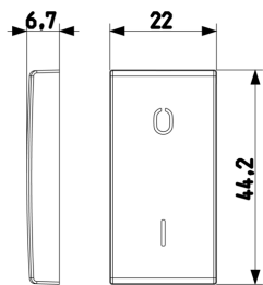
Vista ingombri
