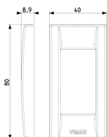
Vista ingombri
