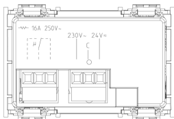
Vista posteriore
