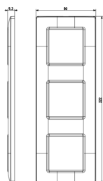
Vista ingombri
