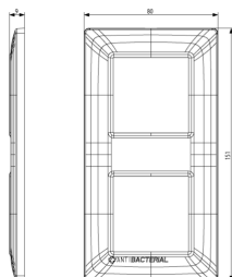
Vista ingombri
