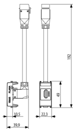
Vista ingombri
