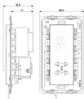
Vista ingombri
