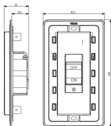
Vista ingombri
