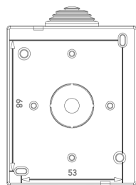
Vista posteriore
