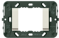
16713 - Supporto 3M +viti 16714 - Supporto 4M +viti 16716 - Supporto 6M +viti 16722.L.B - Supporto 2M liscio scat.inc.3M bianco
