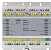
01470.1 - Modulo domotico multifunz. 9in 8out relè
