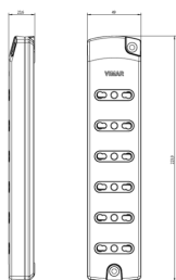
Vista ingombri
