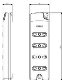
Vista ingombri
