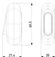
Vista ingombri
