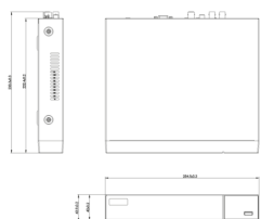
Vista ingombri
