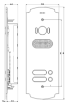
Vista ingombri
