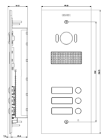
Vista ingombri
