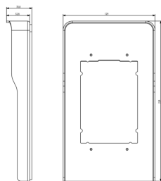
Vista ingombri
