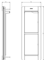
Vista ingombri
