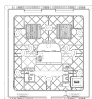
Vista posteriore
