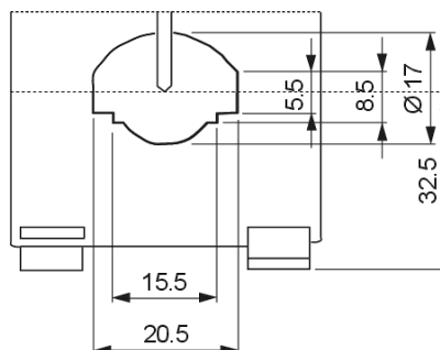
Dettaglio Foro
