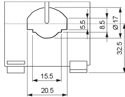
Dettaglio Foro
