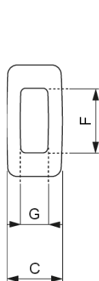
Vista Laterale
