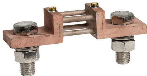
Shunt con portata a 2500 A.
