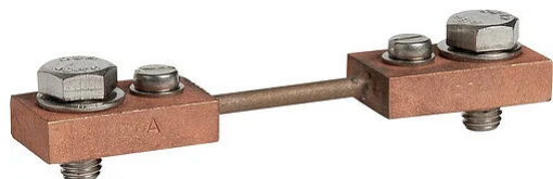
Shunt con portata a 150 A.
