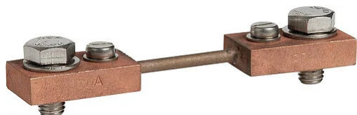
Shunt con portata a 25 A. Con basetta isolante
