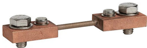
Shunt con portata a 5 A. Con basetta isolante
