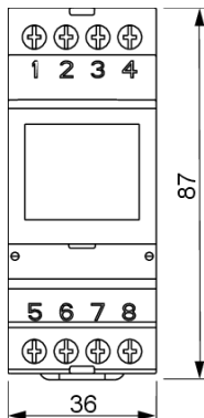
Vista Frontale
