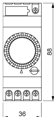
Vista Frontale
