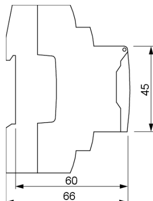
Vista Laterale
