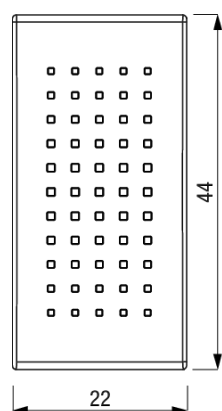
Vista Frontale
