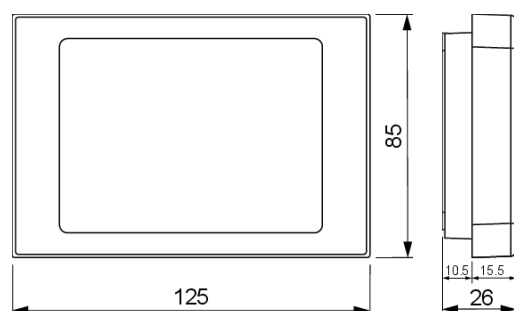
Vista Frontale
