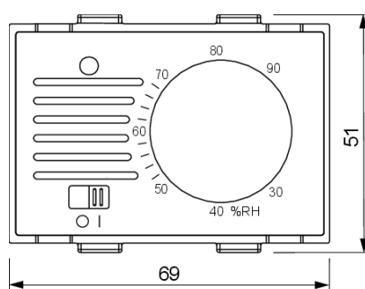
Vista Frontale
