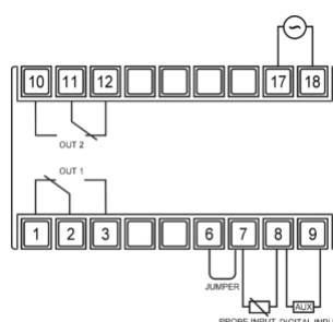
Sonda ingresso PTC 2 fili
