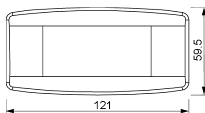
Vista Frontale
