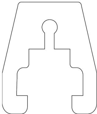
Vista Frontale
