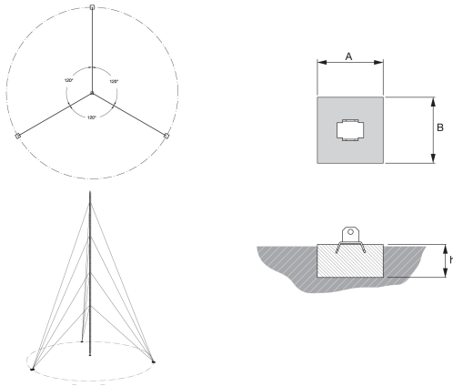
Disegno delle fondamenta della base del traliccio (Nodo centrale) fondamenta dei tiranti (nodo intermedio/esterno).
