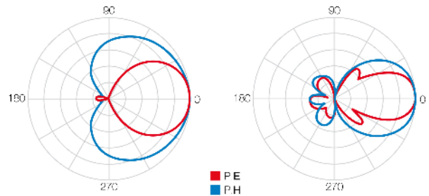
Schema di radiazione
