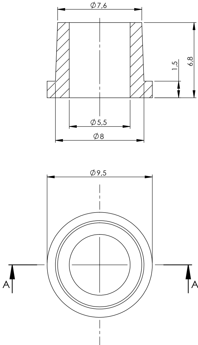
SEZIONE A-A
